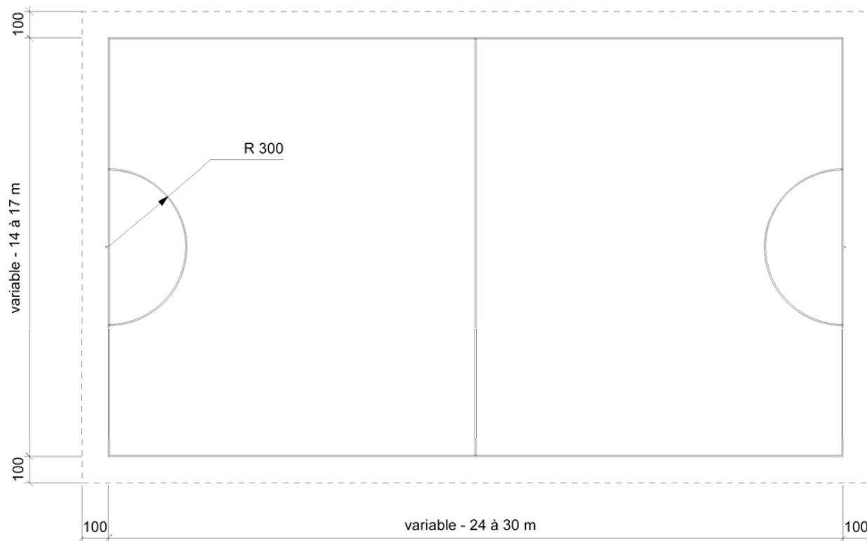
Figure 1 – Dimensions recommandées pour un terrain de taille réduite [cm].
